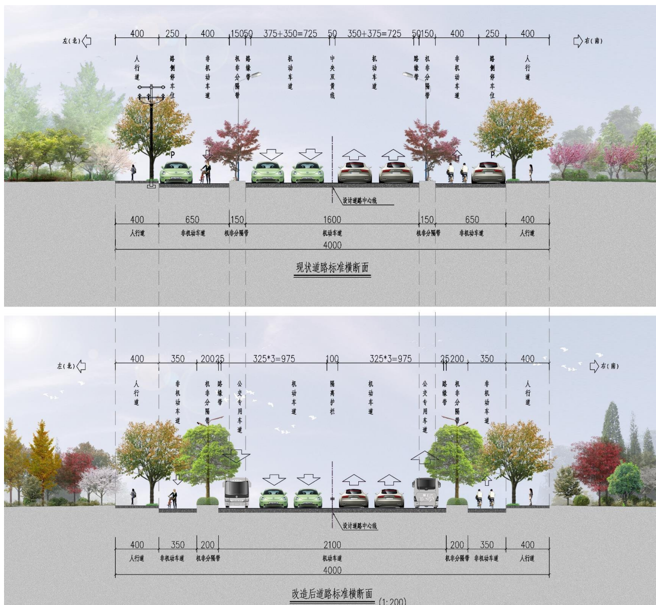
图2.3-1 虹桥路段标准横断面
