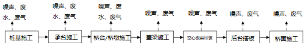
图 8.1-6 桥梁工程施工工艺流程图
